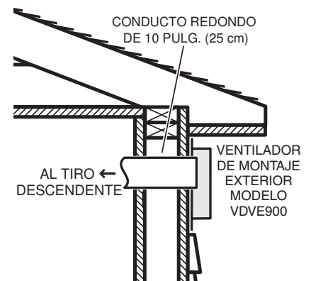
INSTALACIÓN TÍPICA DE MONTAJE EN LA PARED
