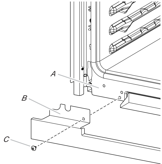
A. Marco del horno B. Lengüeta de ventilación C. Tornillos n.º 8-18 x 3/8" (9,5 mm)
